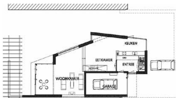
BEGANE GROND VRIJSTAANDE VILLA'S
