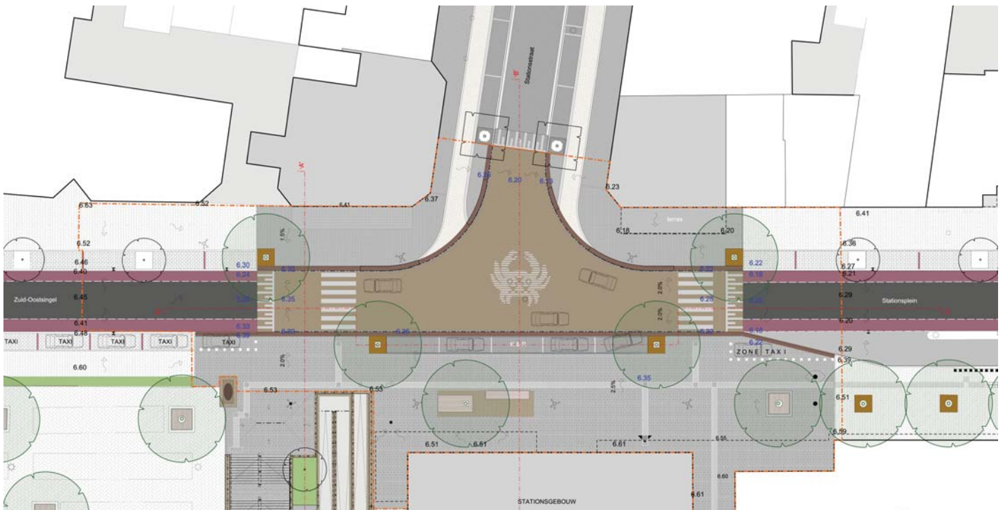
INRICHTINGSPLAN
